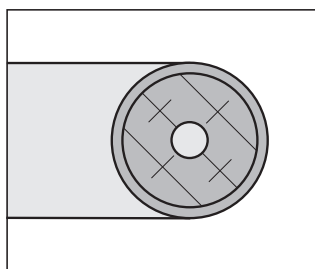
ROK O-Ring mit Hohlkern, nahtlos mit FEP oder PFA ummantelt O-Ring with hollow core, seamless encapsulated with FEP or PFA
